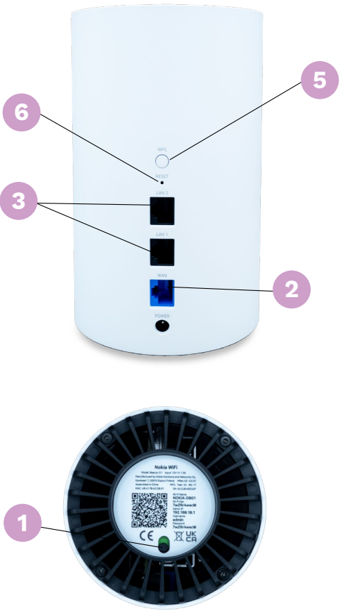
Nokia Beacon 3.1
